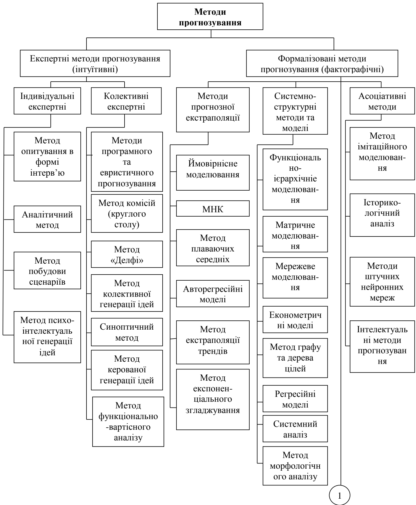
Рис. 1. Сучасна класифікація методів прогнозування
