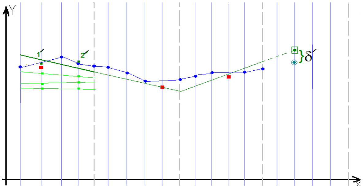
Рис. 5. Етапи роботи алгоритму адаптивного методу плаваючої середньої
