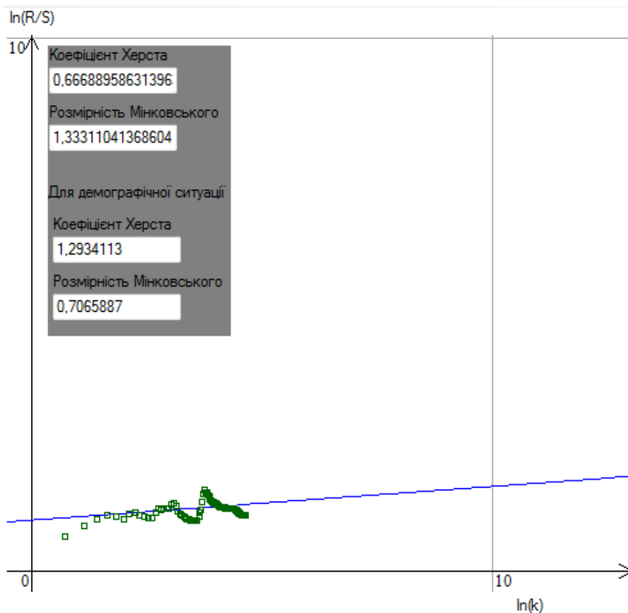
Рис. 3. Приклад розрахунку фрактальної розмірності класичним R/S-методом для соціально-економічних процесів
