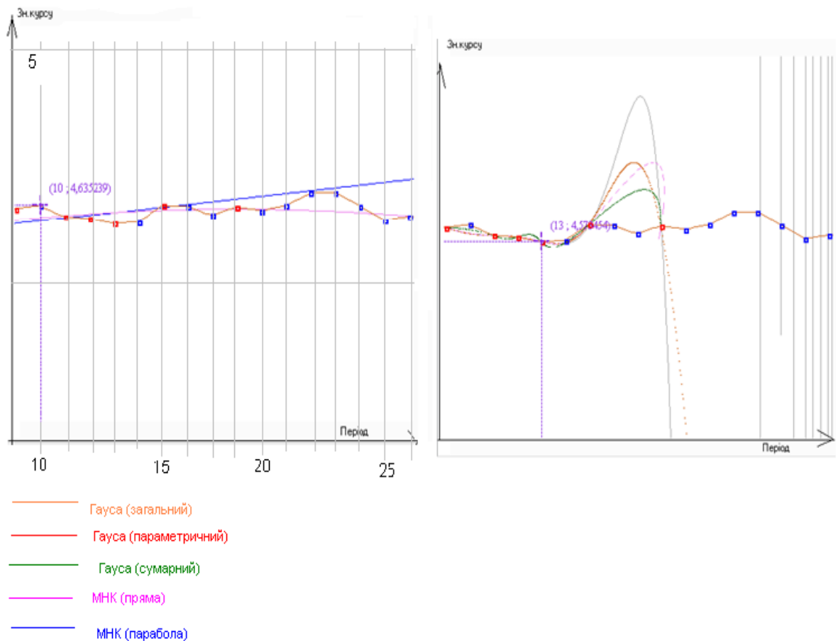
Рис. 4. Результати графічного аналізу класичних методів моделювання
