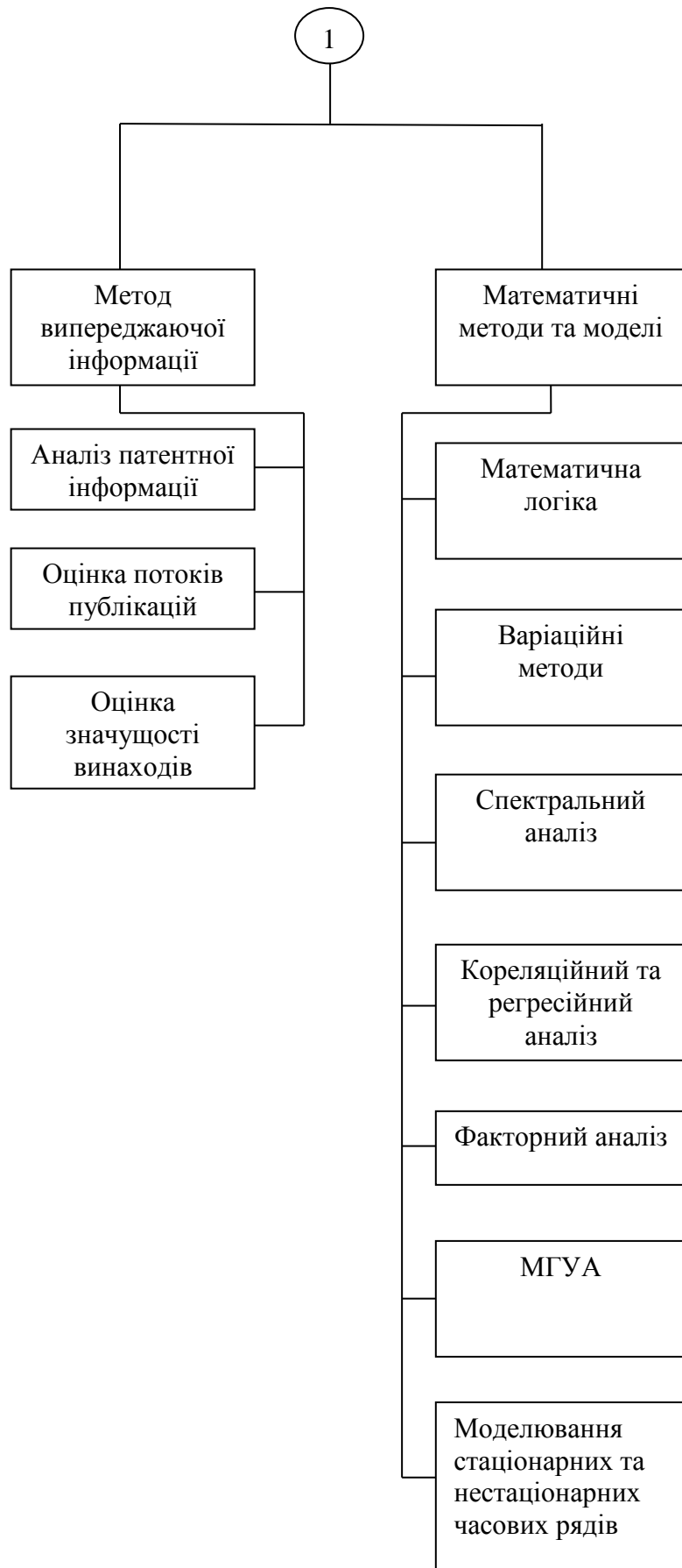
Рис. 2. Сучасна класифікація методів прогнозування
