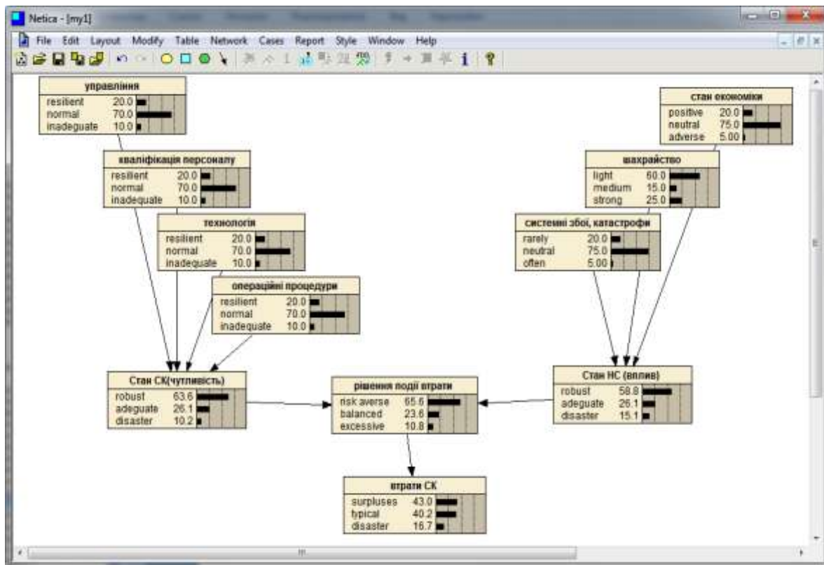
Рис. 5. Байєсівська мережа для аналізу актуарних ОР (NETICA)
